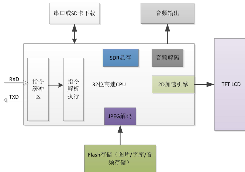
图 7-1M 系列串口屏内部结构图
